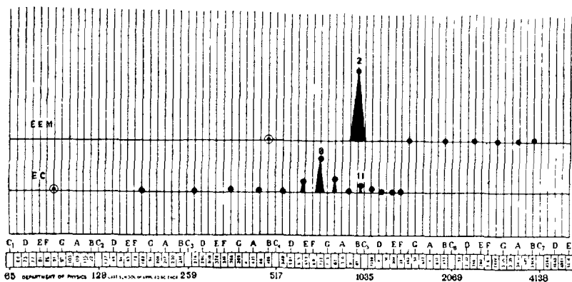
Рис. 7. „Спектры“ голоса сопрано и баса на гласной а .
