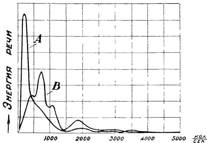
Рис. 12. Распределение энергии в спектре разговорной речи, A — по Крэндаллу и Маккензи, B — по данным Миллера.
