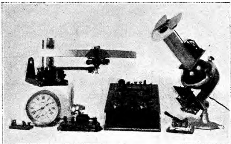
Рис. 2. Пиргелиометр Марвина с принадлежностями.
