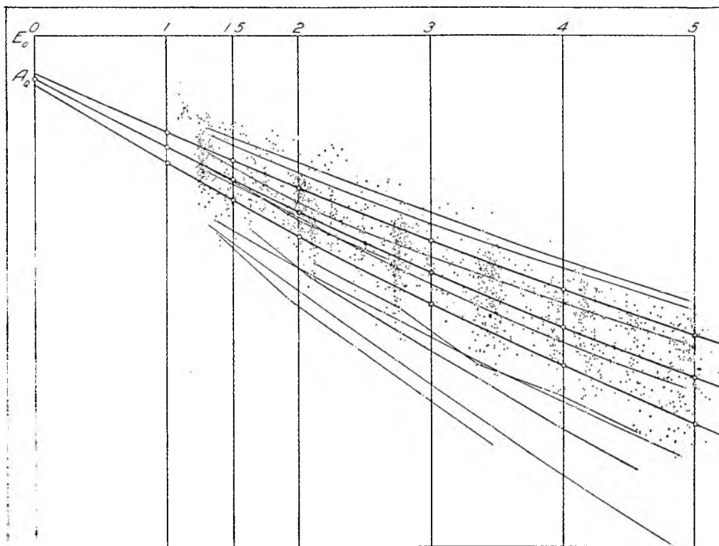
Рис. 19. Рассеяние пиргелиметрических наблюдений в Каламе.
