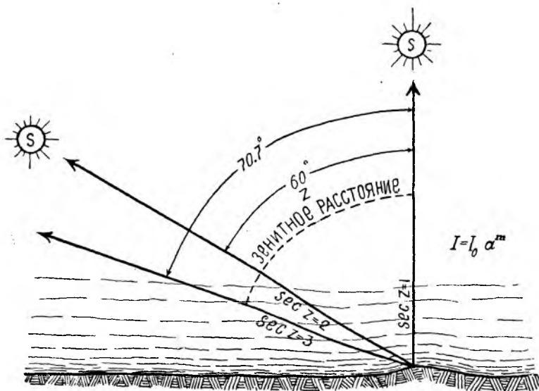
Рис. 9. Изменение «воздушной массы» в различные времена дня, m = \sec z .
