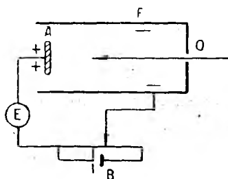
Рис. 3. Монохроматический свет падает через отверстие O на металл A, из которого он вырывает электроны. Кинетическая энергия, с которой эти электроны покидают A, измеряется положительной разностью потенциалов, которую нужно наложить между A и B для того, чтобы ни один электрон не достиг B. Проходящий электронный ток отсчитывается по показаниям E.
