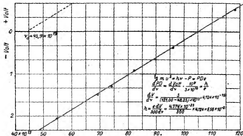
Рис. 5. Рисунок показывает не только то, что между энергией электрона (точки пересечения рис. 4) и действующей частотой света существует линейное соотношение, но в правом нижнем углу также показано, что числовая величина отношения равна 6,56 \cdot 10^{-27} , что хорошо согласуется с другими определениями постоянной Планка h .
