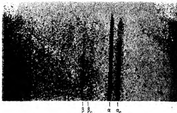
Рис. 6. Эффект Комптона. Этот снимок был сделан Беккером, Смигсом и Уотсоном в апреле 1924 г. На нем видны рентгеновы линии \alpha и \beta , а также линии \alpha_c и \beta_c , соответственно смещенные в красную сторону. Эти последние возникают вследствие столкновения кванта \alpha - и \beta -линий с электронами алюминия. Это важное явление было качественно предсказано А. Комптоном на основании простого допущения, что обычные законы удара справедливы при соударении светового кванта Эйнштейна с электроном. Здесь перед нами новейший успех теории Эйнштейна.
