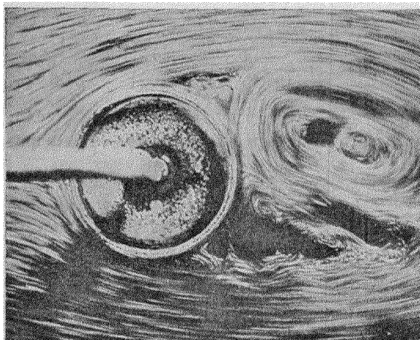
Рис. 21. Образование вихрей около цилиндра. Снимки Рубаха.
