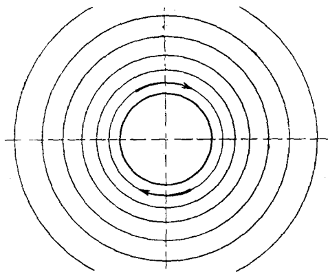
Рис. 4. Циркуляционное обтекание круглого цилиндра.
