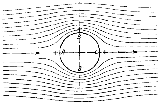
Рис. 3. Потенциальный поток около прямого цилиндра.
