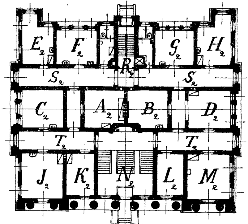
Рис. 9. Первый этажъ.
