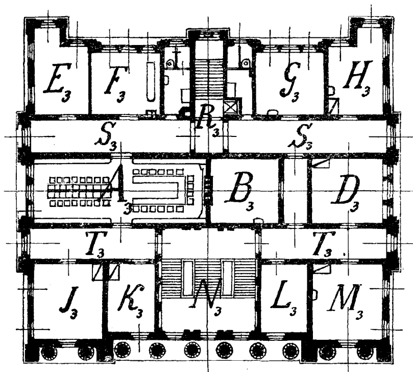
Рис. 10. Второй этажъ.
