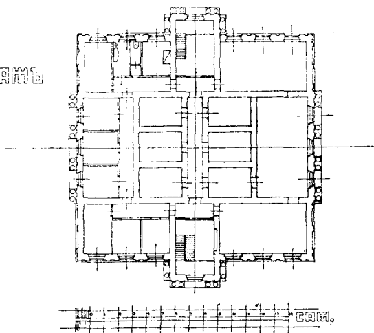
Рис. 4. Первоначальный проект А. Н. Соколова.
