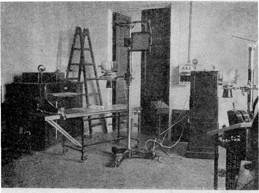
Рис. 19. Рентгеновский кабинетъ.
